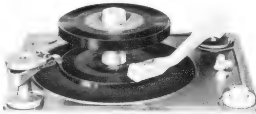
Neuer Dual-Wechsler 1002 F mit dicken Mitteldorn für Kleinplatten
