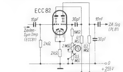
Bild 111. Multivibrator für 15625 Hz
