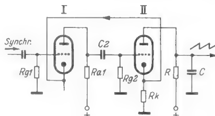
Bild 109. Katodengekoppelter Multivibrator
