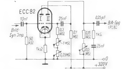
Bild 110. Unsymmetrischer Multivibrator für 50 Hz
