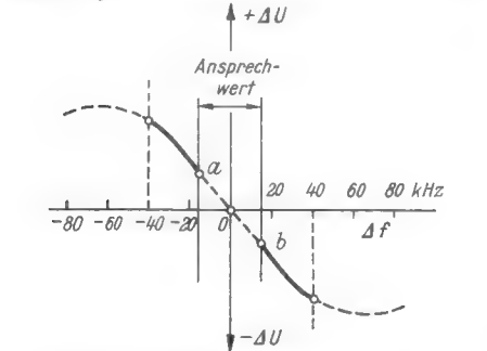
Bild 6. Zahlenmäßige Verhältnisse für die S-Kurve eines Mittelklassengerätes
