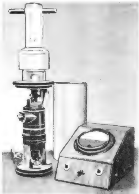
Bild 2. Antennenkopf und Bedienungsteil
