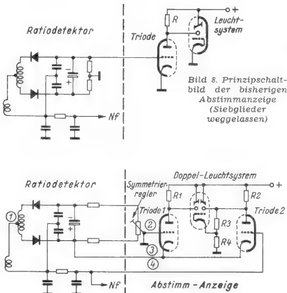
Bild 9. Schaltung für das neue FM-Anzeigeverfahren (Siebglieder und Gittervorspannungserzeugung weggelassen). Die drei Röhrensysteme würde man in einem Kolben anordnen
