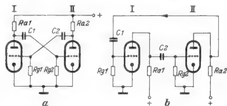
Bild 106. Multivibrator; a = symmetrische Darstellung, b = Darstellung als RC-Verstärker
